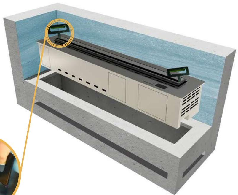
Монтажные держатели
